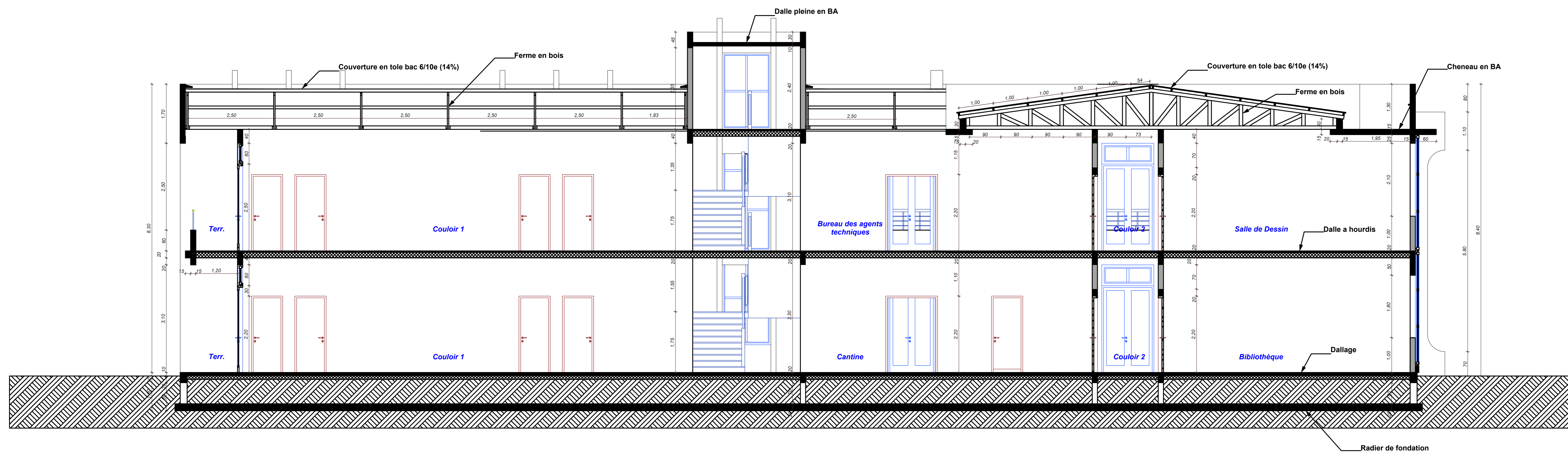
Coupe A-A
