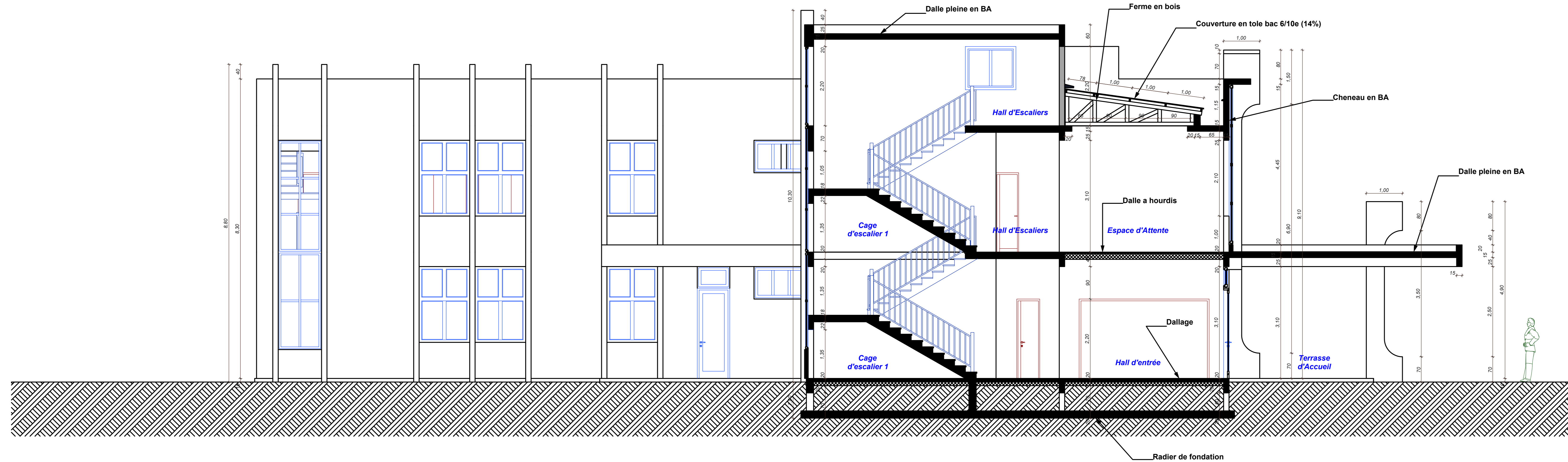
Coupe B-B
