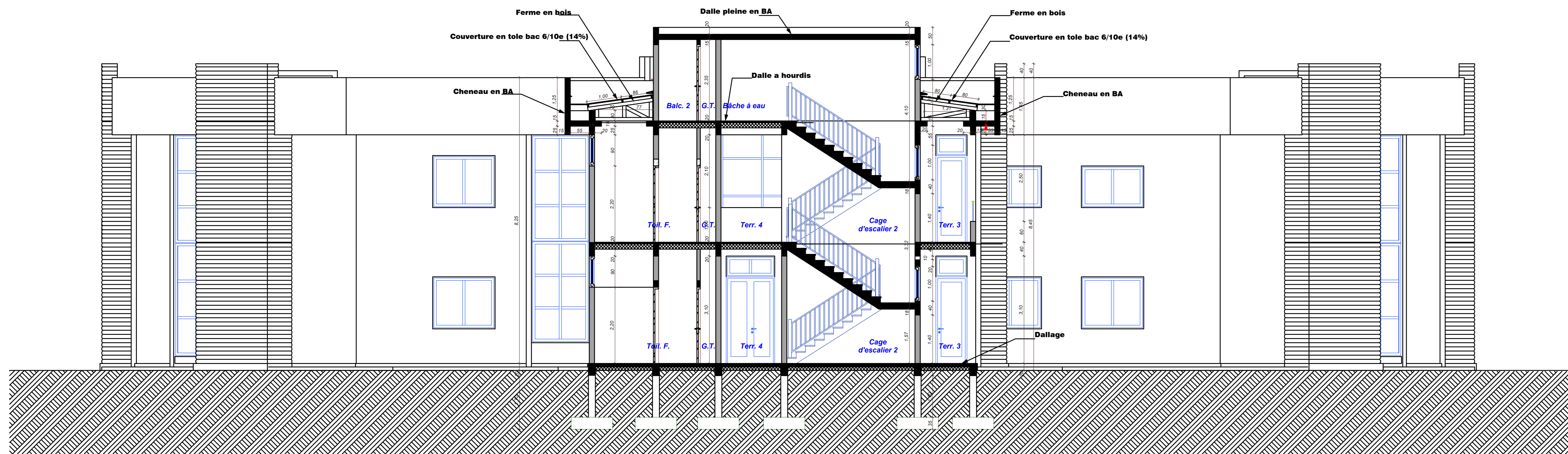
Coupe A-A
