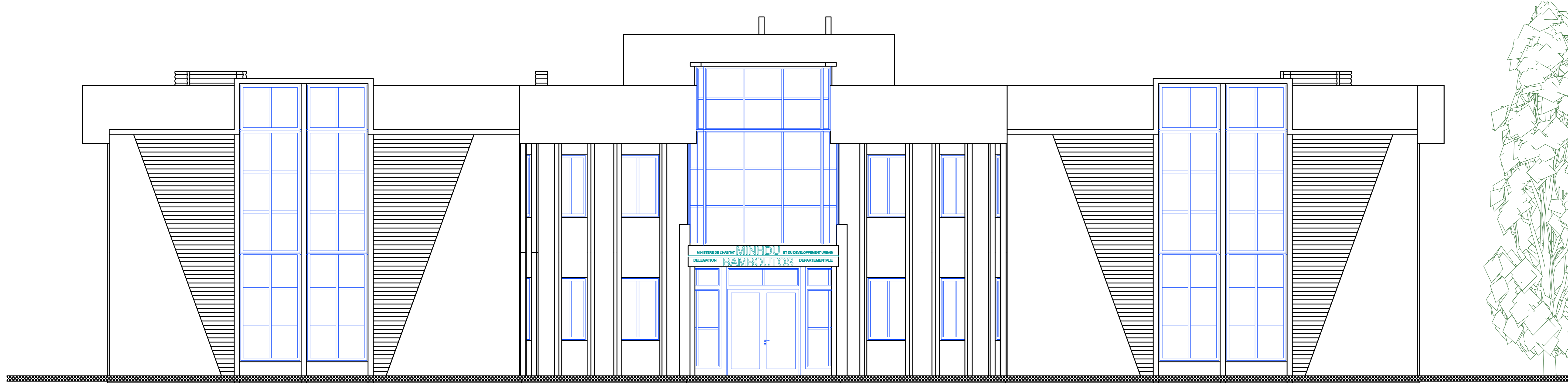
FACADE PRINCIPALE
