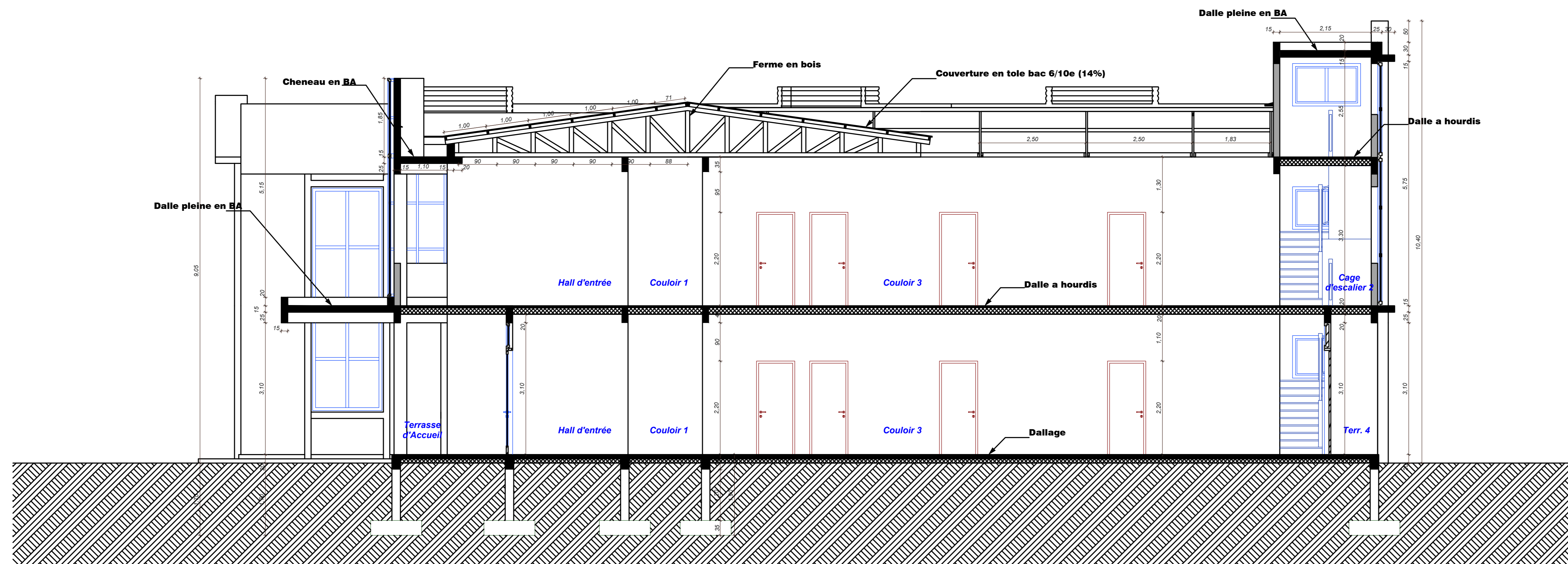
Coupe B-B
